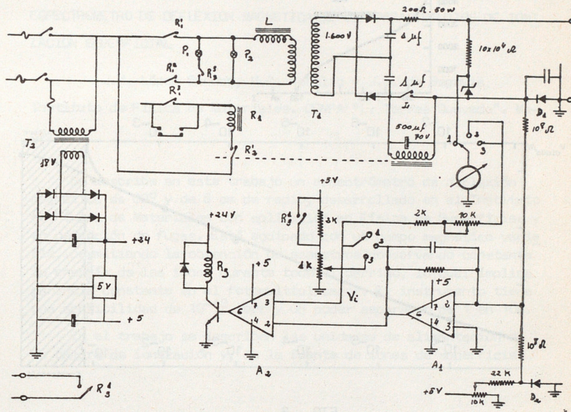
UNIDAD DE ALIMENTACION Y MEDIDA PARA MANOMETRO DE CATODO FRIO
